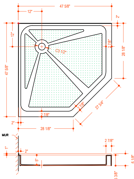
MODÈLE VG06069XXX47
