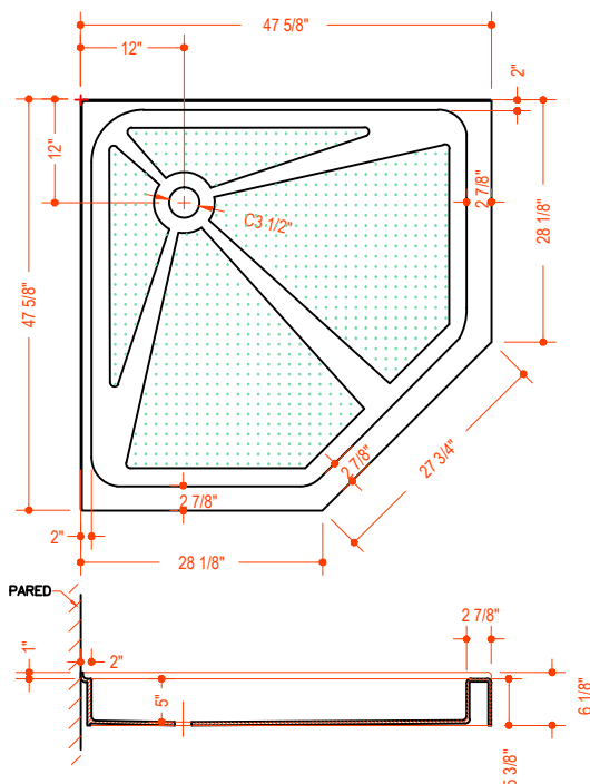
MODELO VG06069XXX47
