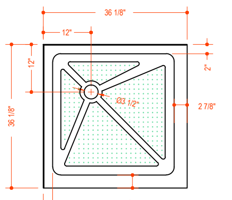
MODÈLE VG06019XXX3240*
