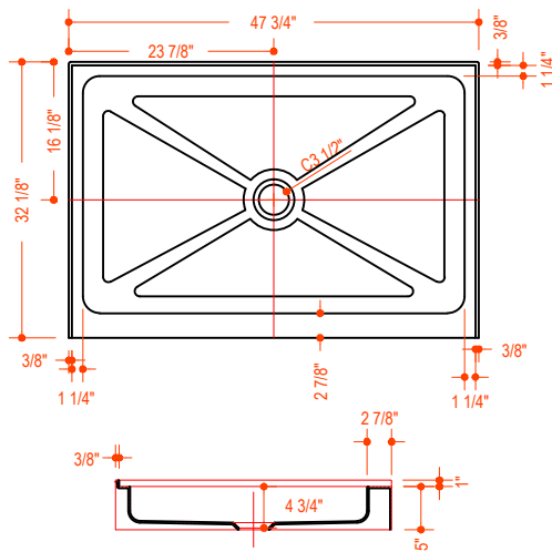
MODELO VG06049XXX4832C
