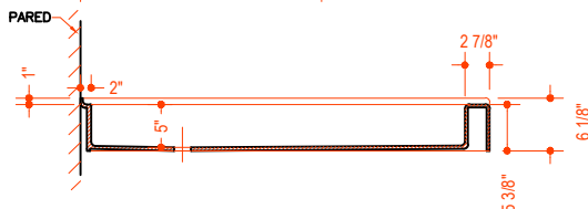
MODELO VG06069XXX47
