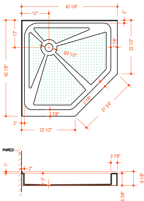
MODELO VG06069XXX42
