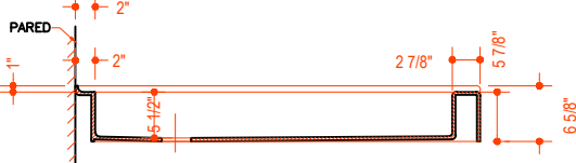
MODELO VG06019XXX3648
