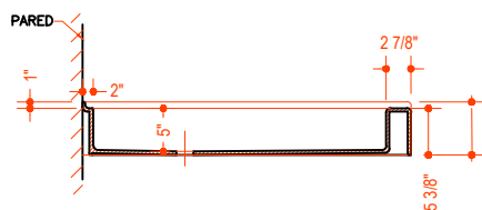
MODELO VG06069XXX38
