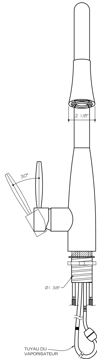
VUE AVANT
