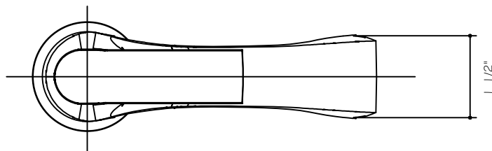
VISTA SUPERIOR
