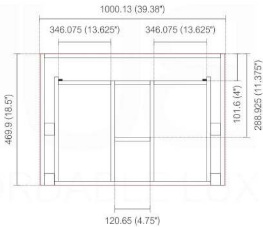
TOP ELEVATION
