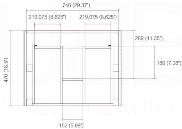
TOP ELEVATION
